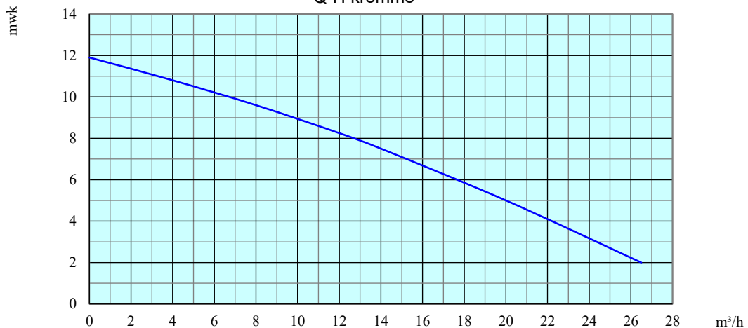
Q-H kromme
