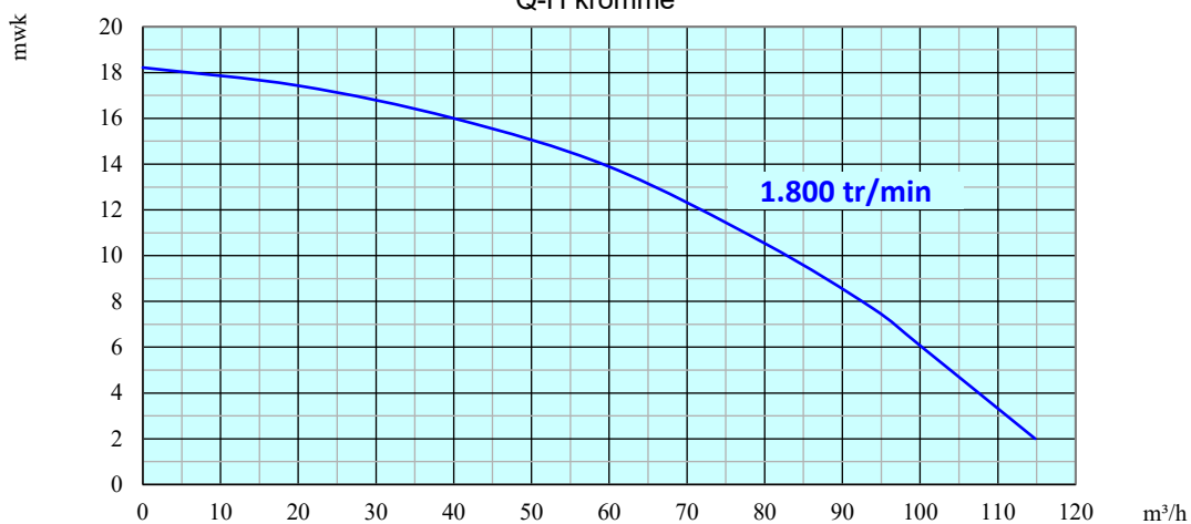
Q-H kromme
