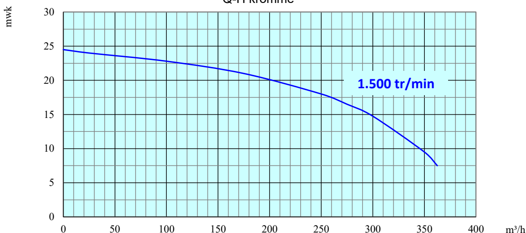
Q-H kromme
