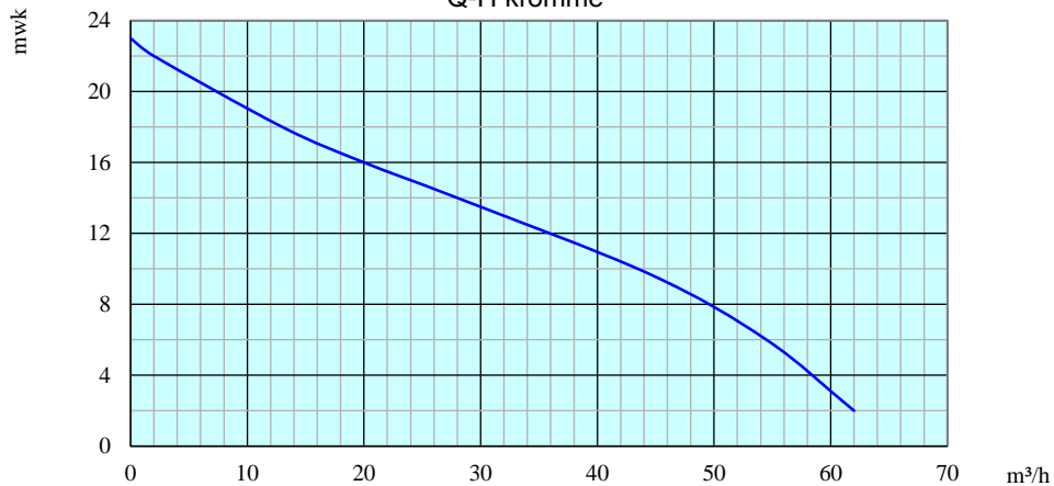
Q-H kromme
