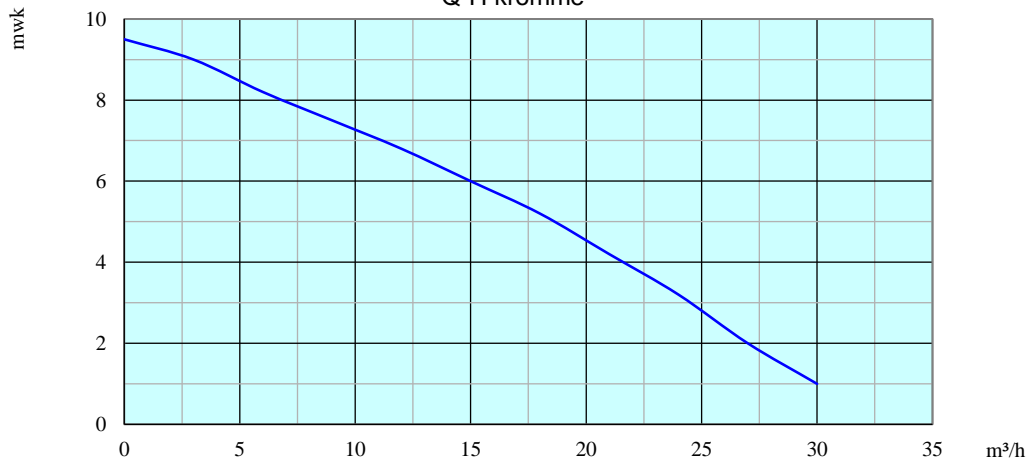
Q-H kromme
