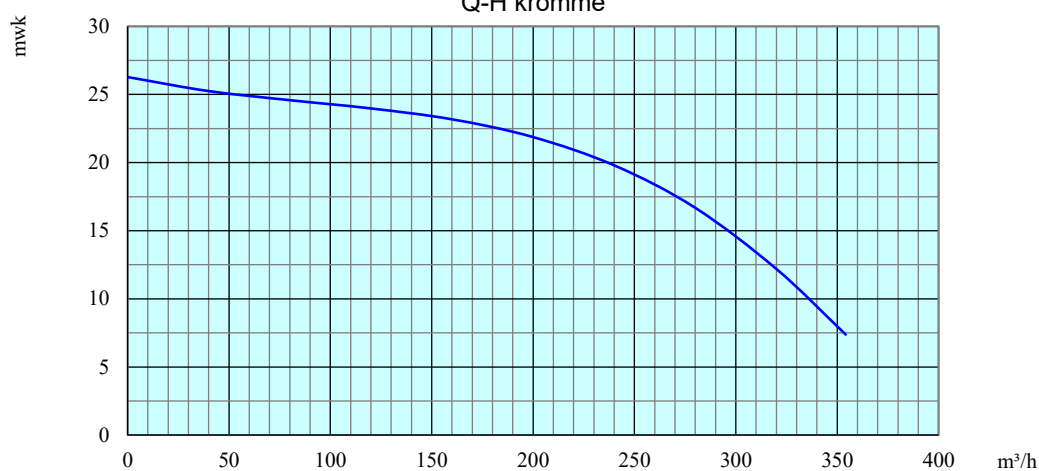
Q-H kromme
