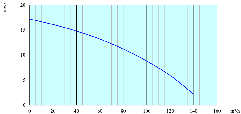
Q-H kromme
