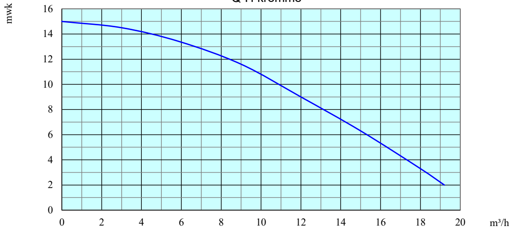
Q-H kromme
