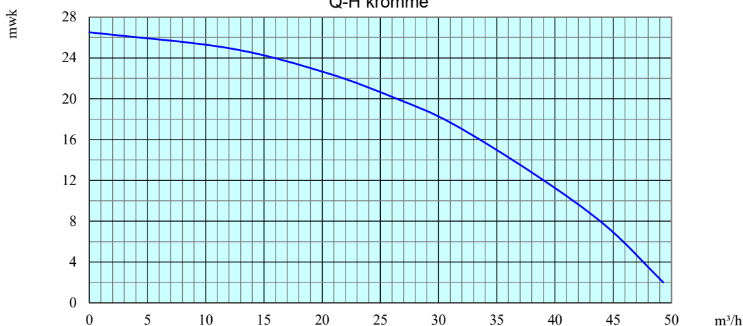
Q-H kromme
