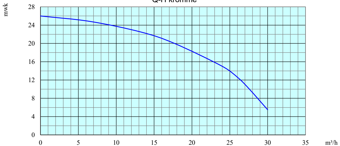
Q-H kromme
