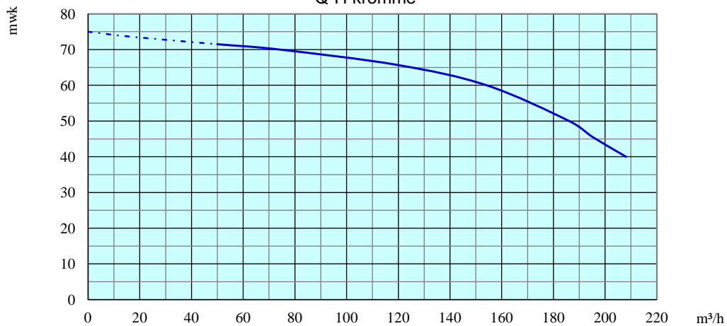
Q-H kromme
