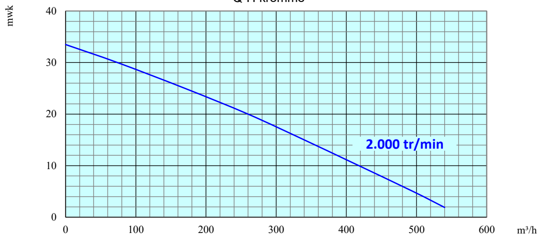
Q-H kromme
