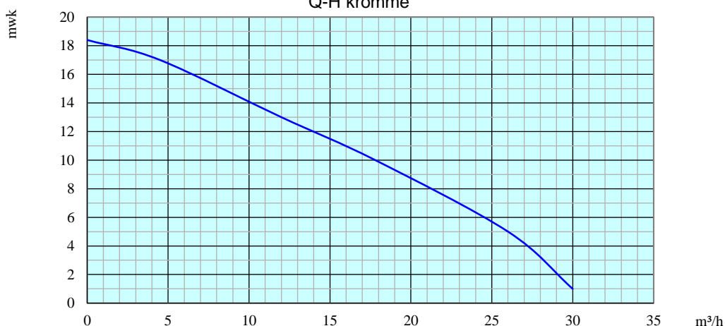
Q-H kromme
